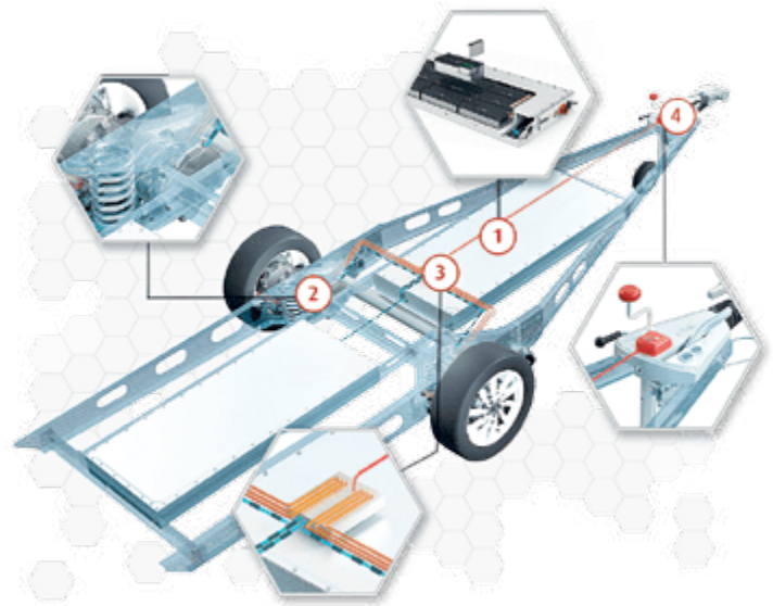
Schema Dethleffs Coco elektrische aandrijving
